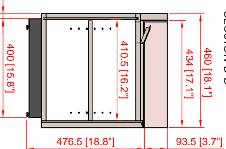
SECCIÓN B-B'
