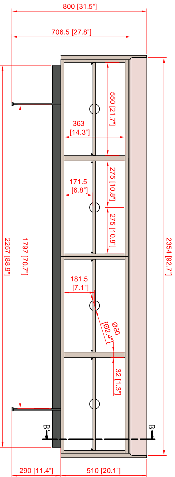
SECCIÓN A-A'
