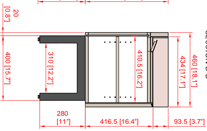
SECCIÓN B-B'
