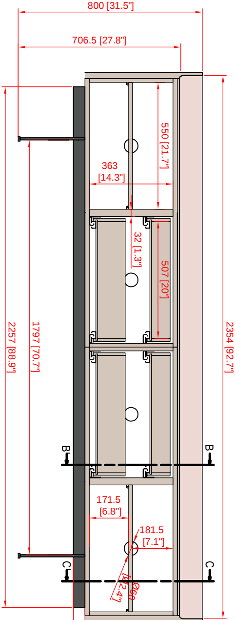
SECCIÓN A-A'
