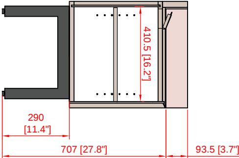
SECCIÓN C-C'
