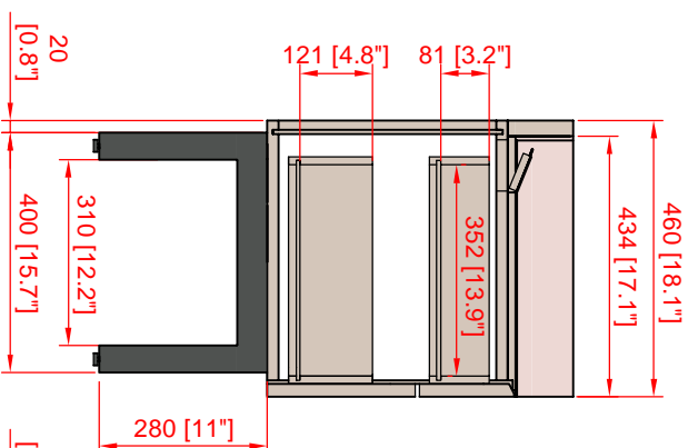
SECCIÓN B-B'
