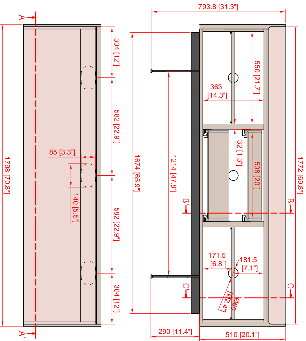
SECCIÓN A-A'
